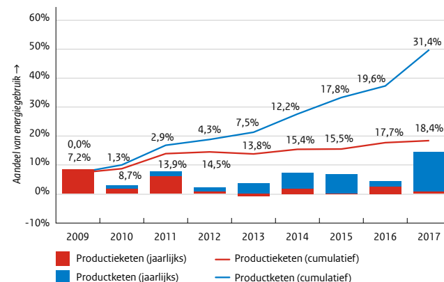
Figuur 2.8 – Besparing door ketenefficiëntie MEE-convenant (referentiejaar 2009; PJ)
